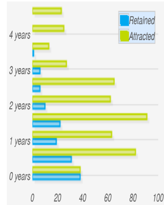
CloudStack
